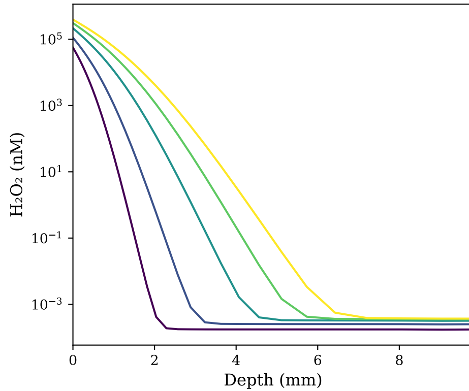
(d) \text{H}_2\text{O}_2
