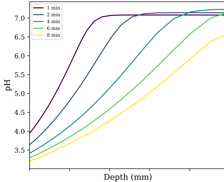
(d) \text{H}_2\text{O}_2
